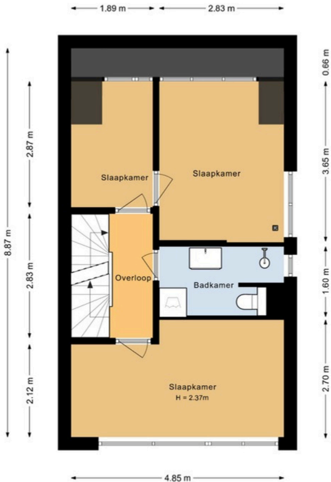
De Krommert 62 Eerste verdieping
