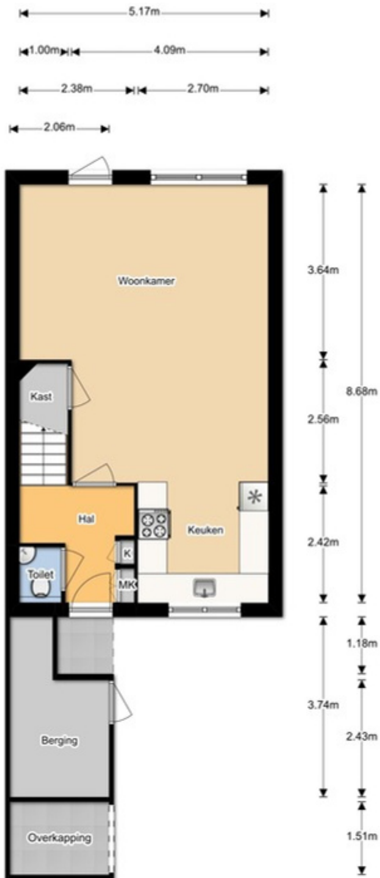
Begane grond
