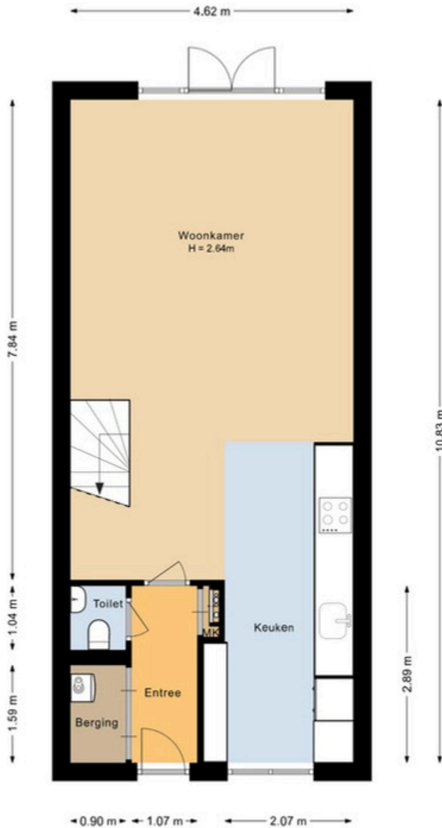
Kraaiennest 7, 1474 MW, Oosthuizen Begane Grond
