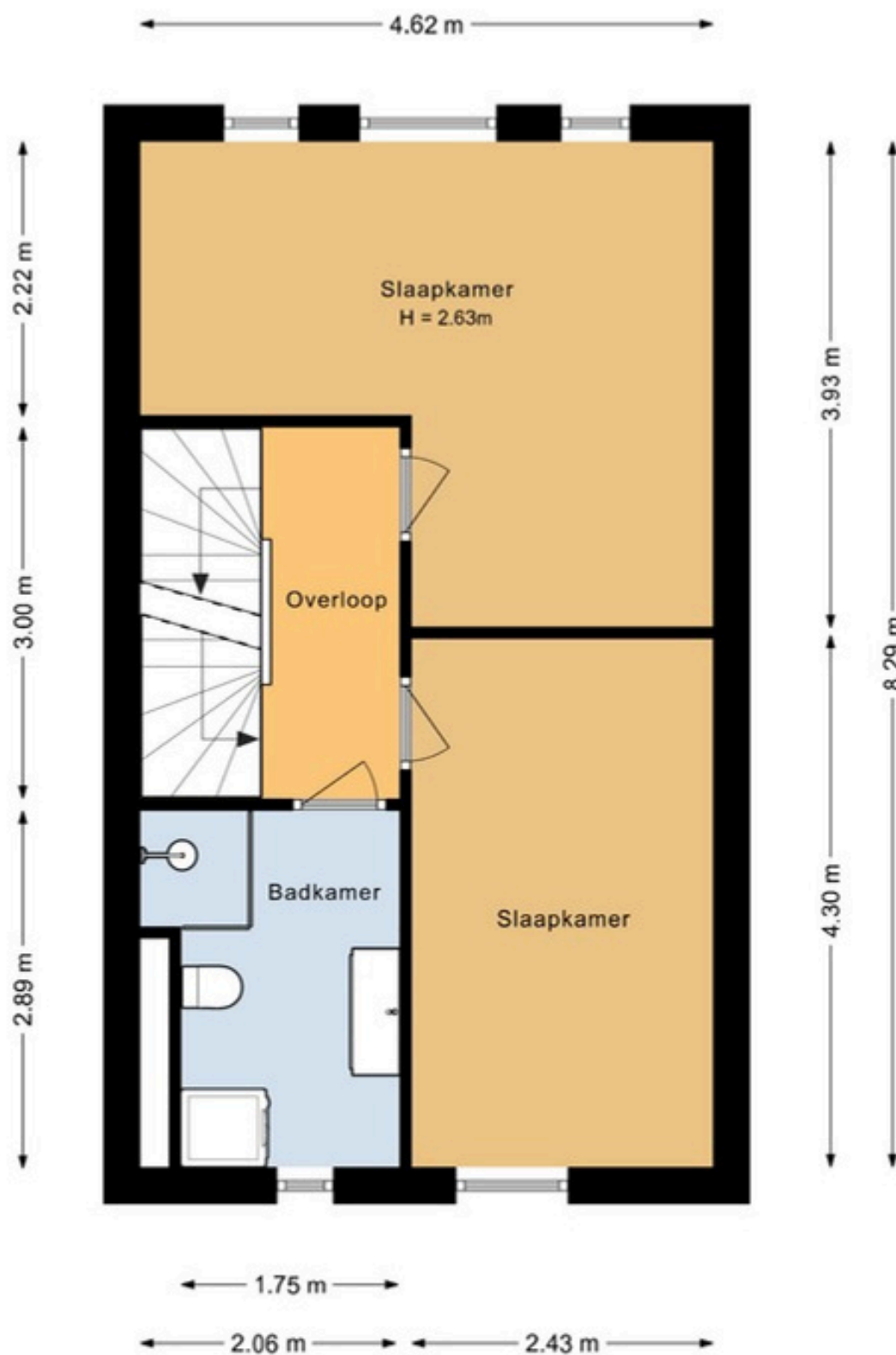
Kraaiennest 7, 1474 MW, Oosthuizen Eerste verdieping
